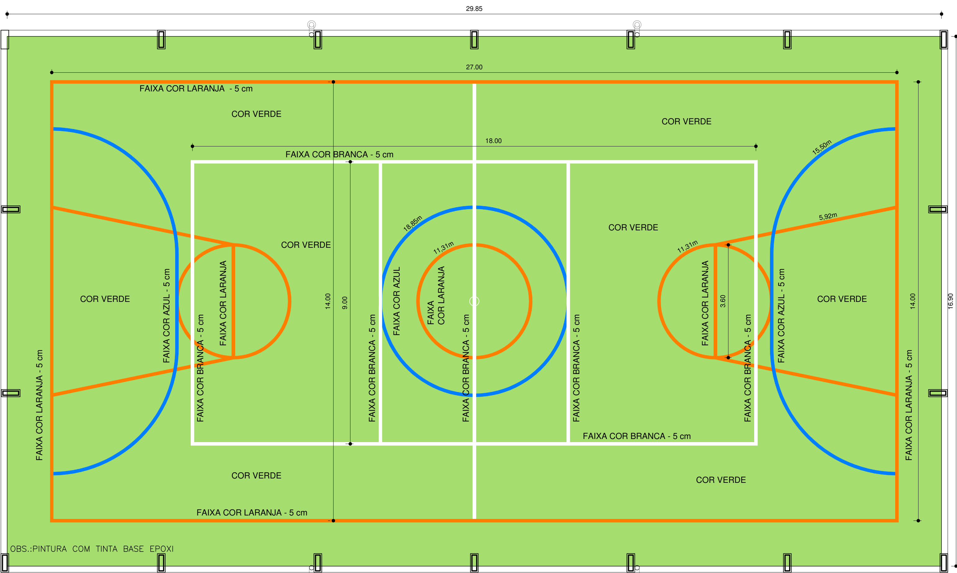
PLANTA-BAIXA Escala: 1/75
